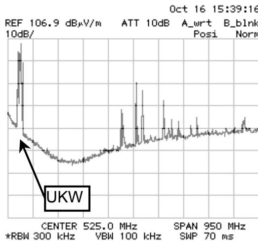
Abbildung 3: Übersichtsmessung 50 bis 1000 MHz, horizontale Polarisation
