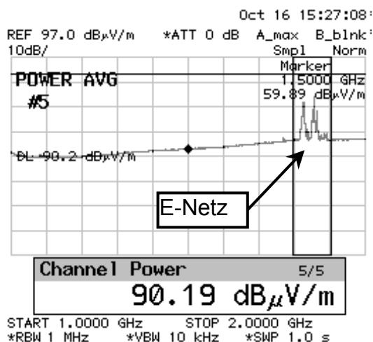
Abbildung 5: Übersichtsmessung 1000 bis 2000 MHz, vertikale Polarisation
