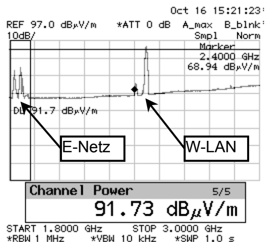
Abbildung 6: Übersichtsmessung 1800 bis 3000 MHz, vertikale Polarisation
