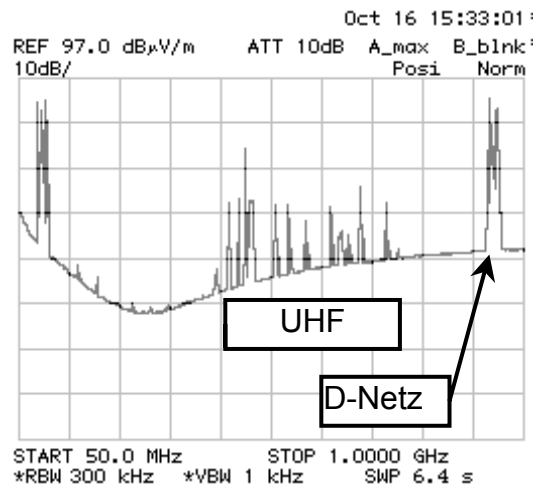
Abbildung 4: Übersichtsmessung 50 bis 1000 MHz, vertikale Polarisation
