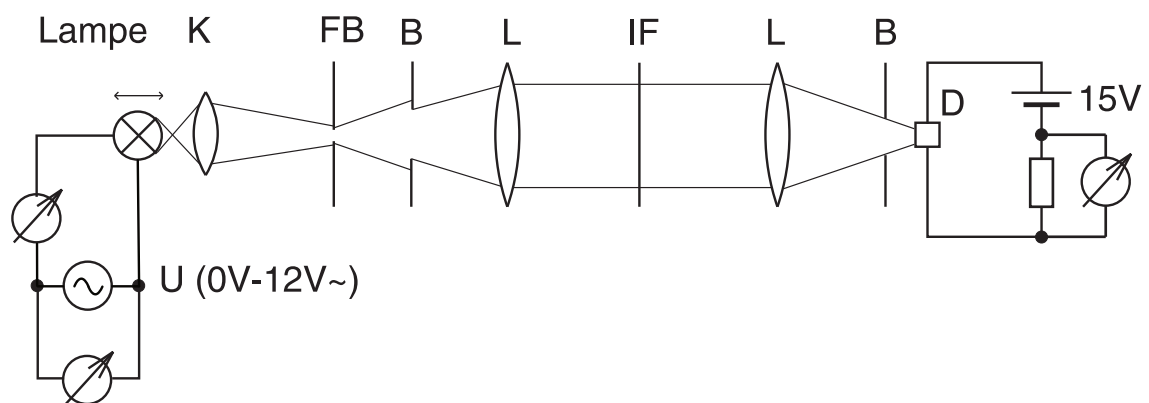
Abbildung 2: Aufbau zur Messung der Intensität eines grauen Strahlers.
