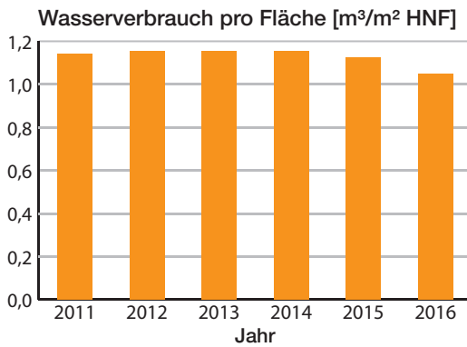
Spezifischer Wasserverbrauch pro Hauptnutzfläche [HNF]
